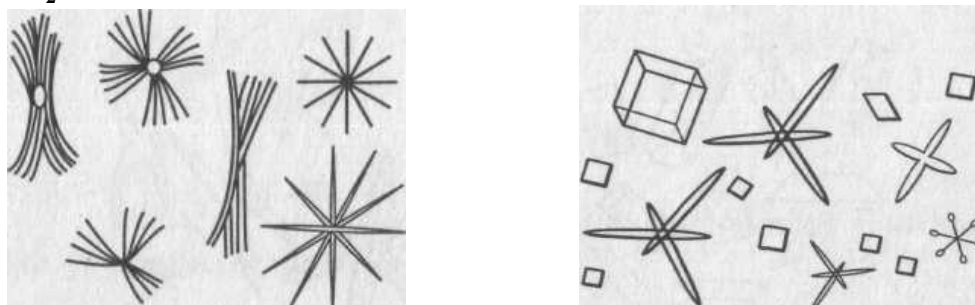
Рис. 5. Кристаллы фосфата ртути (а) и фосфат-молибдата аммония (б)
